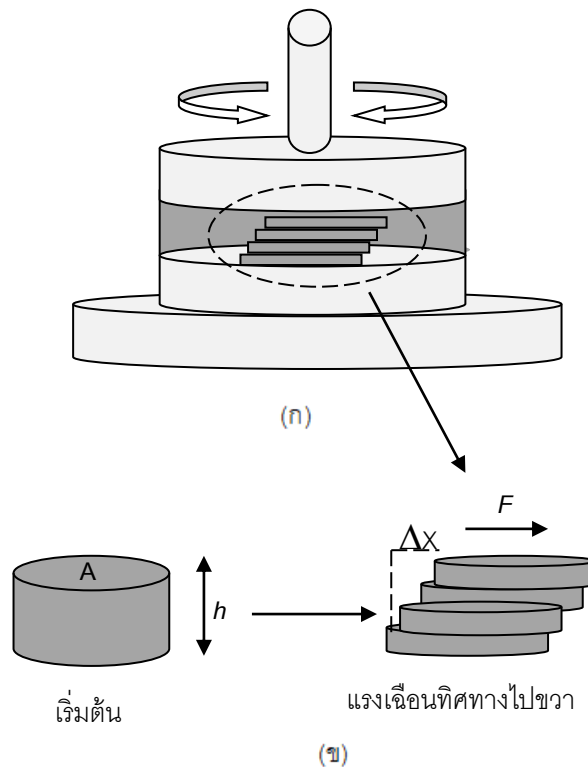
ภาพที่ 2 การสั่นเฉือนพลาวัต (ก) การวางตัวอย่างบนแผ่นเรียบที่ประกบด้านบนบนด้วยทรงกระบอก และ (ข) แรงบิดเฉือนไปทางด้านขวา
