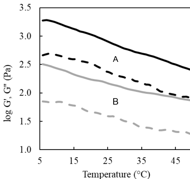
ภาพที่ 9 เทมเพอร์เจอร์สวีฟ ผลิตภัณฑ์โยเกิร์ตสองยี่ห้อ คือ ยี่ห้อ A (เส้นสีดำ) และยี่ห้อ B (เส้นสีเทา): (—) ค่ามอดูลัสยืดหยุ่น และ (-----) มอดูลัสหนืด วัดค่าที่ร้อยละเสียดสภาพ 0.5 ความถี่เชิงมุม 100 เรเดียน ต่อ วินาที ช่องว่างตัวอย่าง 1 มิลลิเมตร
